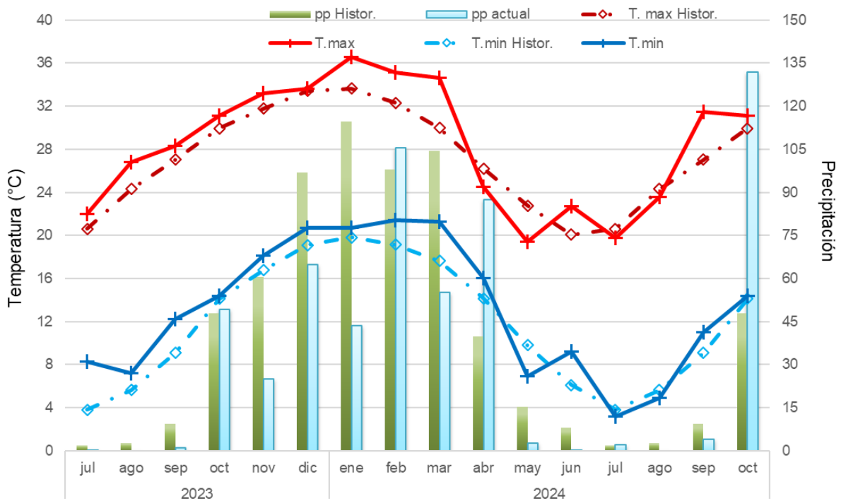
Figura 1. Temperatura máxima promedio mensual y mínima promedio mensual y precipitaciones mensuales y promedio histórico entre julio a noviembre 2024, para el Campo Experimental Francisco Cantos, INTA Santiago del Estero. Fuente: Ing. Agr. Nelson Dominguez. dominguez.nelson@inta.gob.ar .
